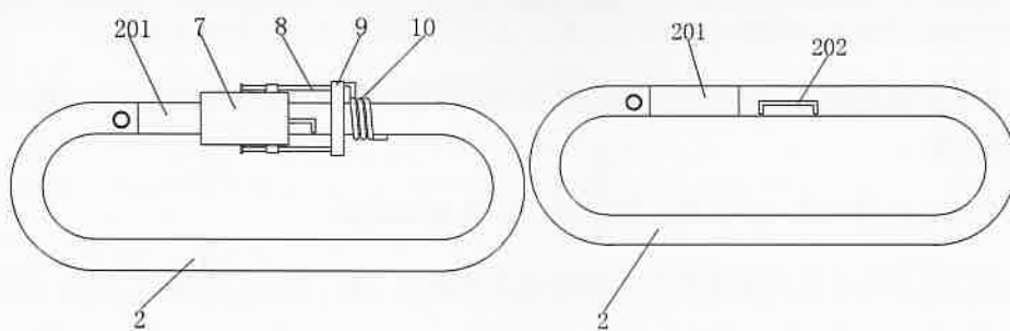
201、翻转轴; 202、槽孔; 7、套筒; 701、导向套; 8、导向杆; 9、转盘; 10、扭簧
