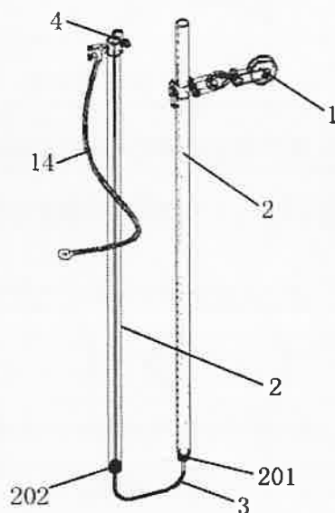
1、滑轮；2、直管；201、外螺纹；202、内螺纹；3、钢索；4、螺栓；14、绳索
