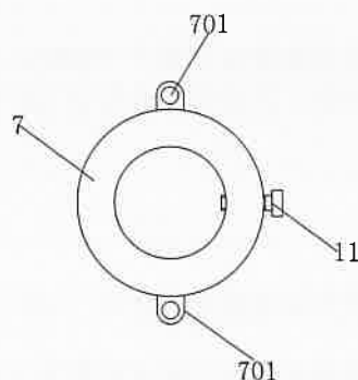
图 4 安全扣环的锁扣套筒结构示意图
