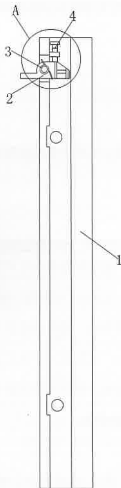
1、导轨；2、挡板；3、弹性件；4、螺栓
